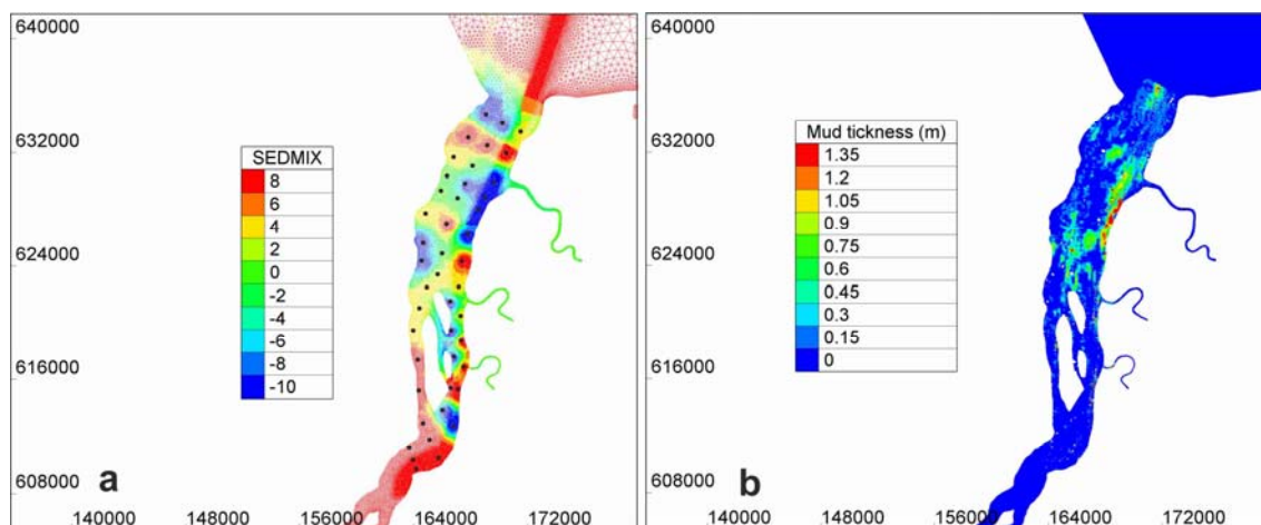
Figure 2. a) Carte des sédiments superficiels, obtenue par interpolation sur une grille TELEMAC (rouge : sable, vert : vase consolidée ; bleu : vase fluide). Les points indiquent la localisation des prélèvements sédimentaires. b) Carte d'épaisseur de vase détectée à l'échosondeur.
